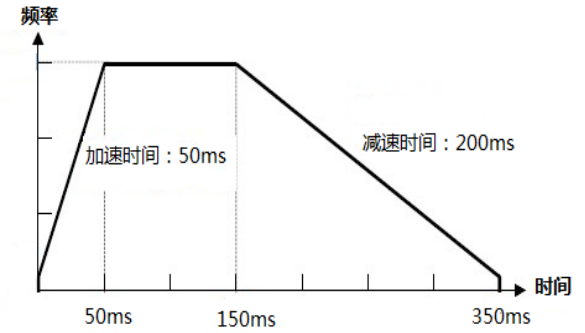
图 1 非对称梯形曲线加减速
