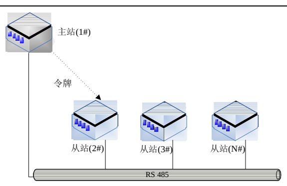
图10-4 主站向2#从站发放令牌
