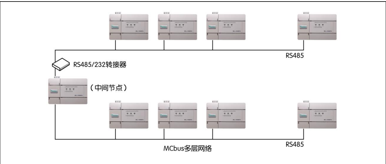
图10-2 MCBus 多层网络
