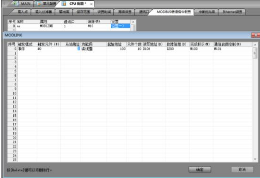
RS485 modbus 便捷指令配置
