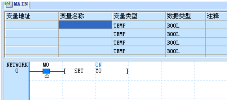
图2-20 被强制软元件的锁标记
