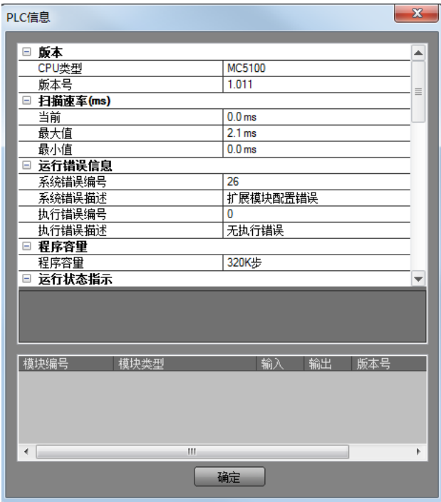
图2-16 PLC 当前运行信息
