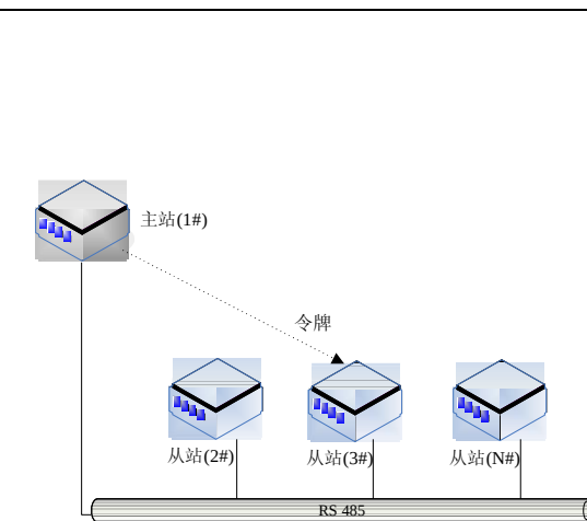
图10-6 主站向3#从站发放令牌
