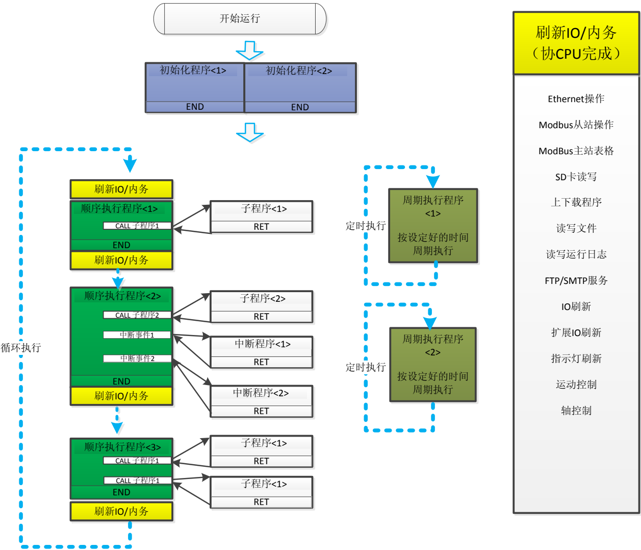
图 2.1 PLC 运行机制
