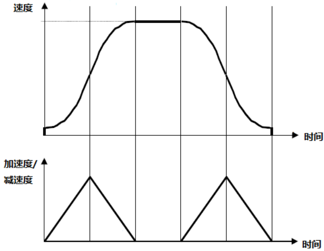
图 2 对称 S 形曲线加减速
