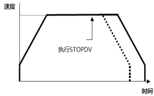
图 1 剩余距离大于减速距离
