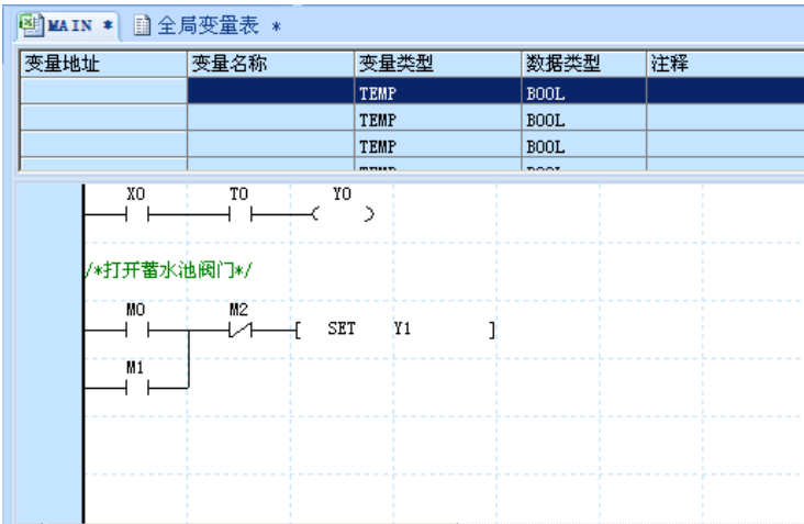
图4-8 未选中符号编址的状态
