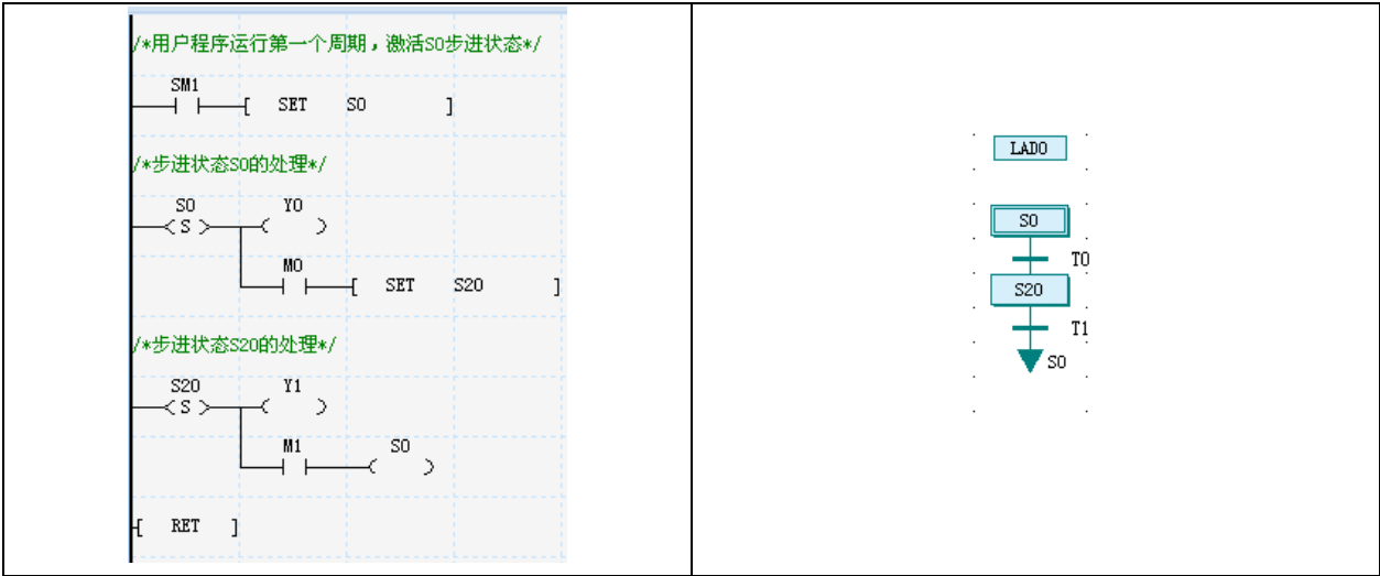
图4-3 顺序功能图示例
