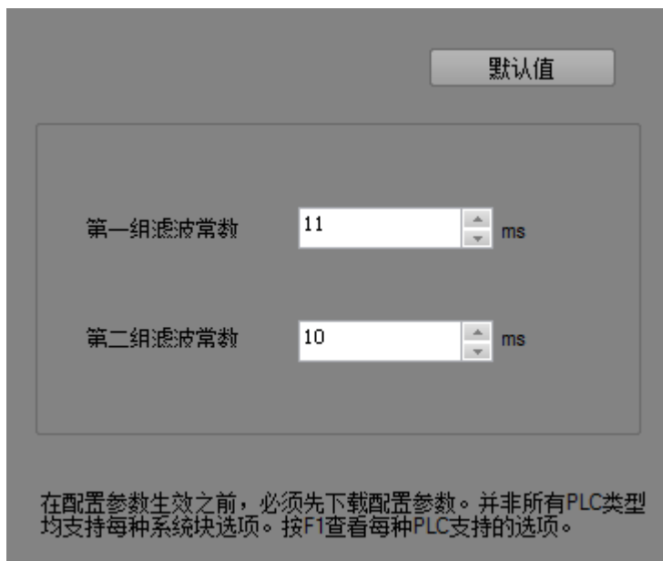
图2-6 设置输入过滤器
