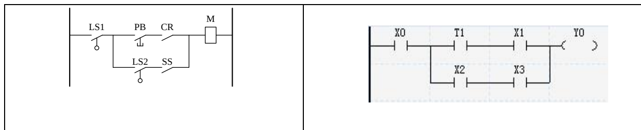
图4-1 电气控制图和梯形图的等效关系
